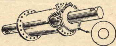
Fig. 3 - Il perno della pedivella verrà reso solidale al mozzo della moto saldandolo in sede.
