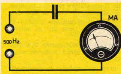
Fig. 1 - Un condensatore si lascia attraversare da una tensione alternata proporzionalmente alla frequenza applicata
